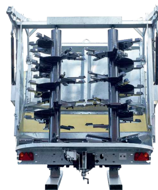
Szórószerkezet kidobólapáttal
