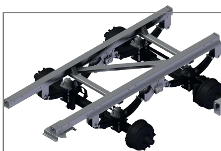
»Gigant« tandem futómű (TMK 200 5,65 m teknőhossztól)
