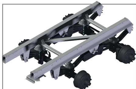
»Gigant Plus« futóműrugózás
