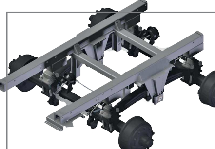
»Titan« tandem futómű a legjobb talajkiegyenlítésért
