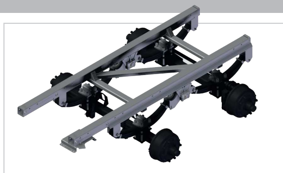
Gigant tandem futómű - parabolarugózás
