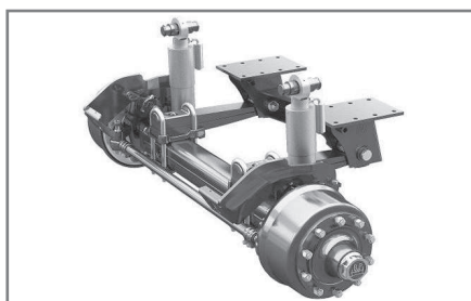
Hidraulikus rugózás
