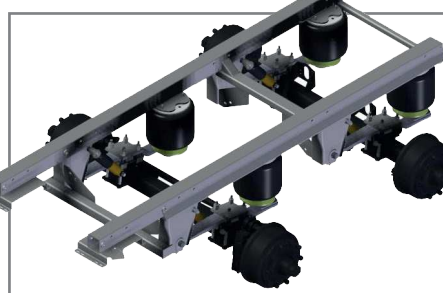
Légrugózás
