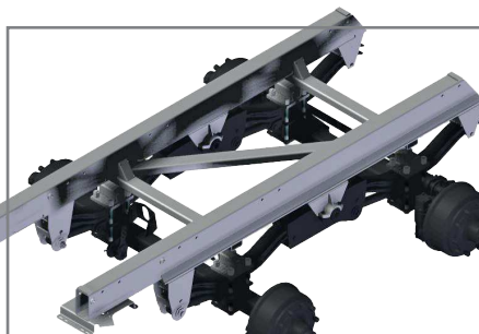
»Gigant Plus« tandem futómű
