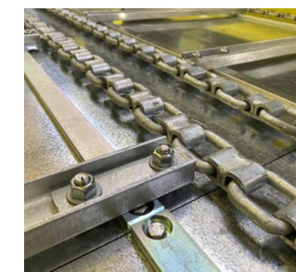
Verschraubter Kratzboden mit verzinkten Leisten
