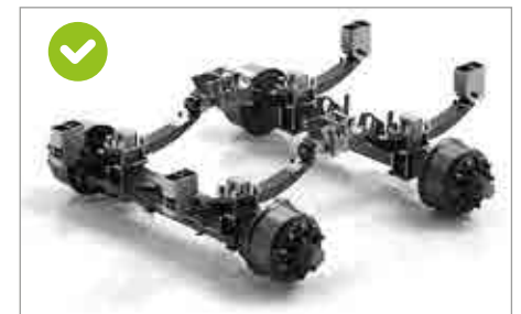
Tandemaggregat Gigant bei 11000 L, 12500 L und 14000 L POLY Line Plus
