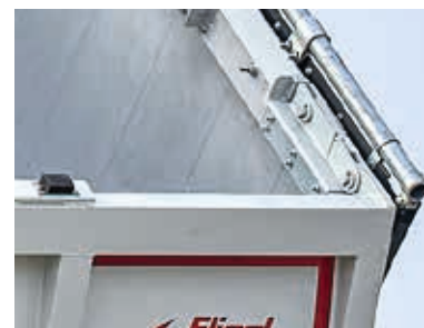
Dvojitý kloubový závěs a 2násobné hákové zajištění
