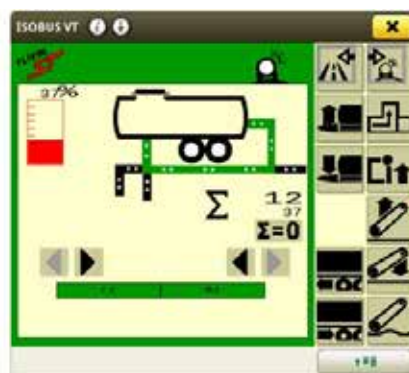
Gebruikersinterface FST Bedieningsmodus veld
