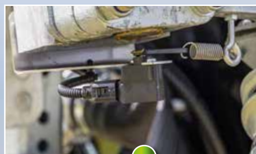
Hoeksensoren links en rechts voor gelijkmatig uit- en inklappen op een helling
