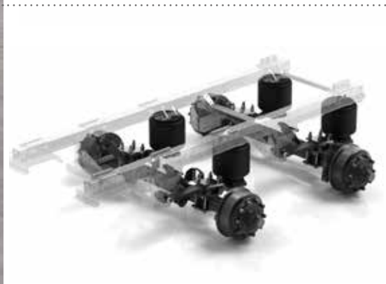
Luchtvering
